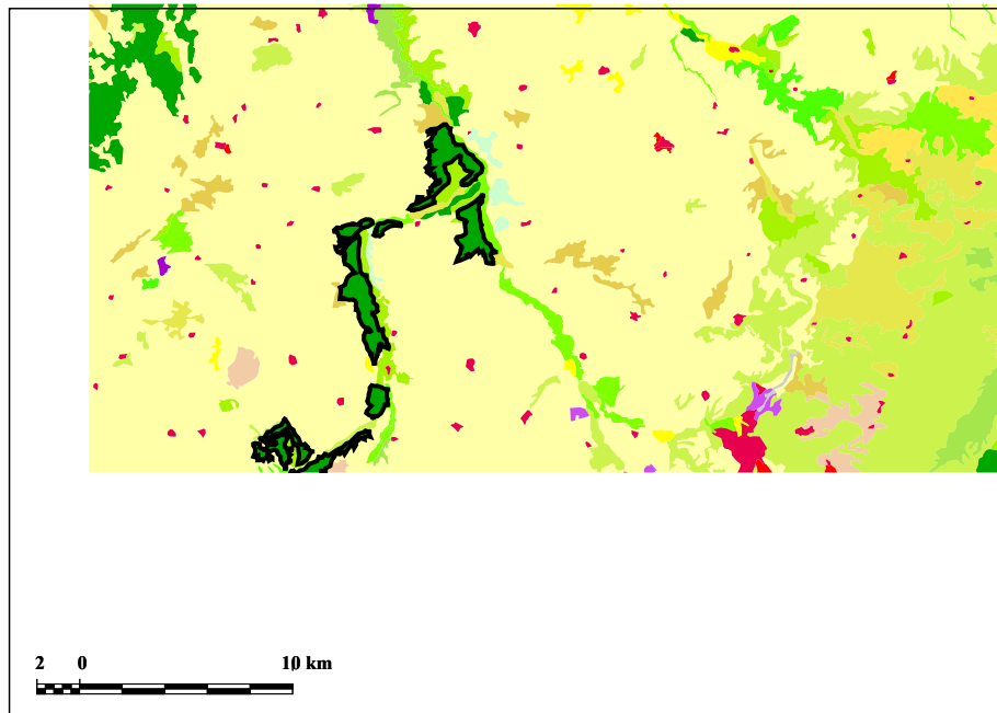
Figura 4.6. Zona de estudio, con los pinares de estudio marcados con un reborde negro. Fuente: CORINE Land cover Map, 2000.
