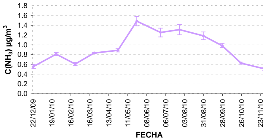
Figura 21: Concentraciones de Amoniac (NH 3 µg/m 3 ) entre durante el año 2010 en la parcela de Villanueva de la Sierra.
