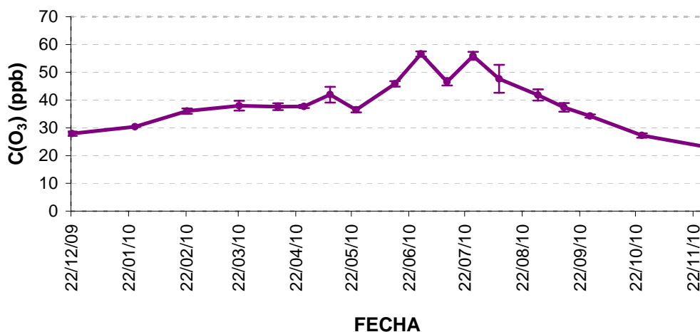
Figura 18: Concentraciones promedio de ozono (ppb) en el año 2010 en la parcela de Villanueva de la Sierra.
