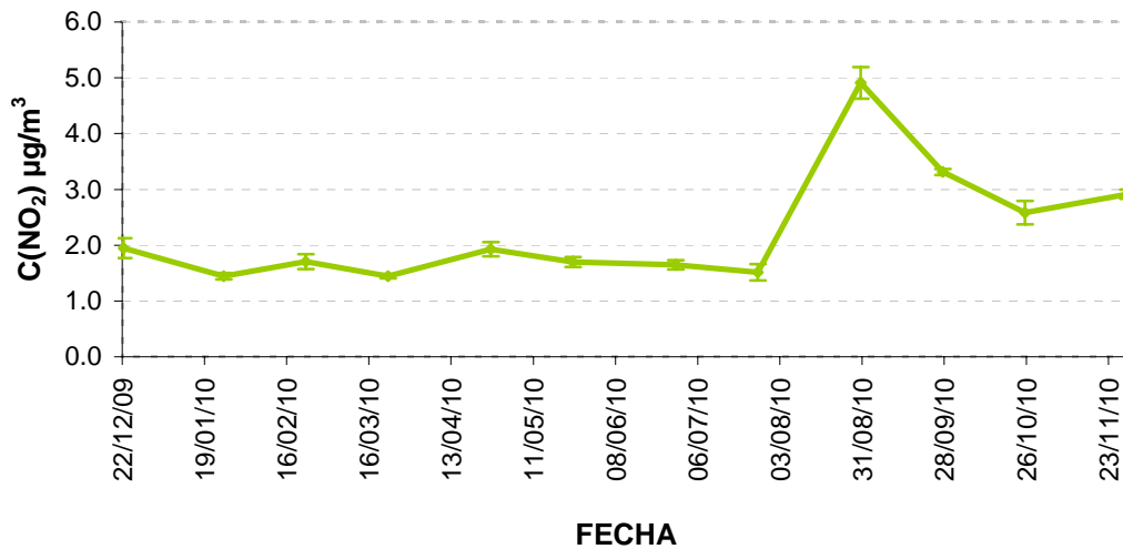
Figura 19: Concentraciones de Dióxido de Nitrógeno (NO 2 µg/m 3 ) en el año 2010 en la parcela de Villanueva de la Sierra.
