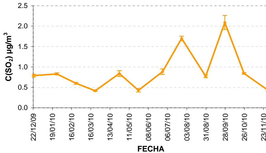
Figura 20: Concentraciones de Dióxido de Azufre (SO 2 µg/m 3 ) durante el año 2010 en la parcela de Villanueva de la Sierra.
