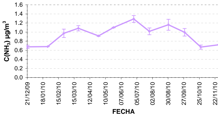
Figura 25: Concentraciones de Amoniac (NH 3 µg/m 3 ) entre durante el año 2010 en la parcela de Burguete.
