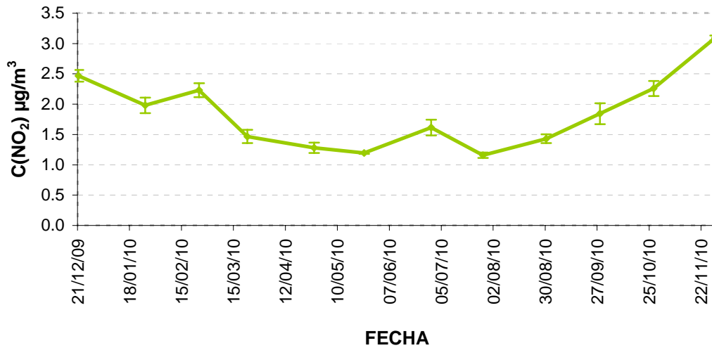
Figura 23: Concentraciones de Dióxido de Nitrógeno (NO 2 µg/m 3 ) en el año 2010 en la parcela de Burguete.
