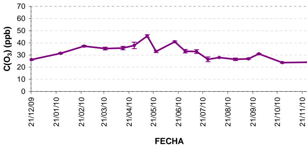
Figura 22: Concentraciones de ozono (ppb) en el año 2010 en la parcela de Burguete.
