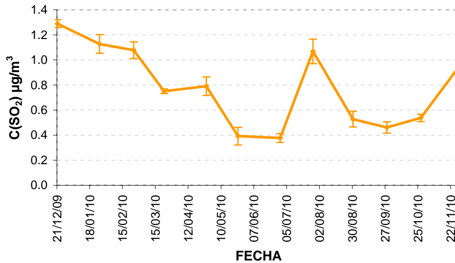
Figura 24: Concentraciones de Dióxido de Azufre (SO 2 µg/m 3 ) durante el año 2010 en la parcela de Burguete.
