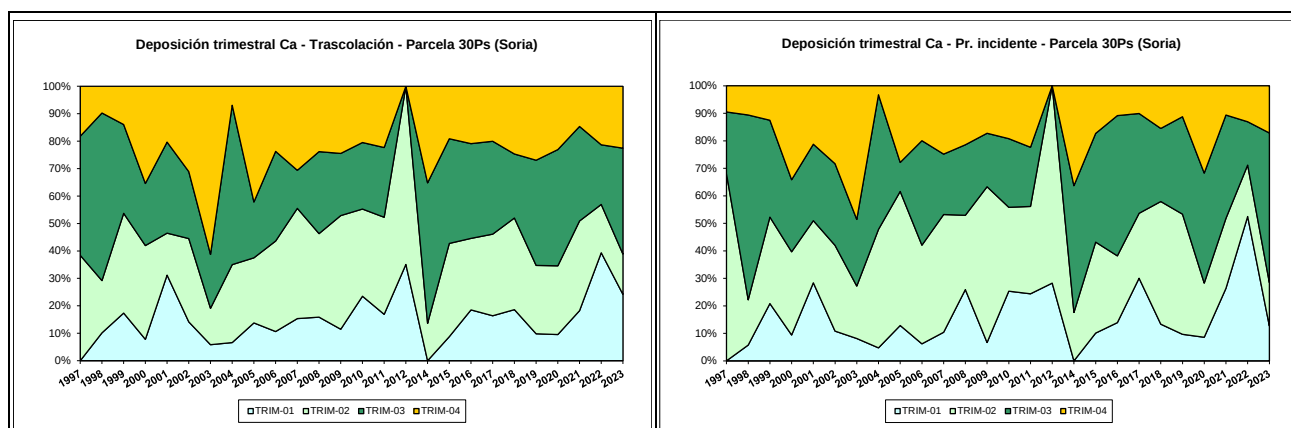
FIG 11: Variación temporal de deposición de Ca, diferencia TR-PI, porcentaje de deposición por trimestres
