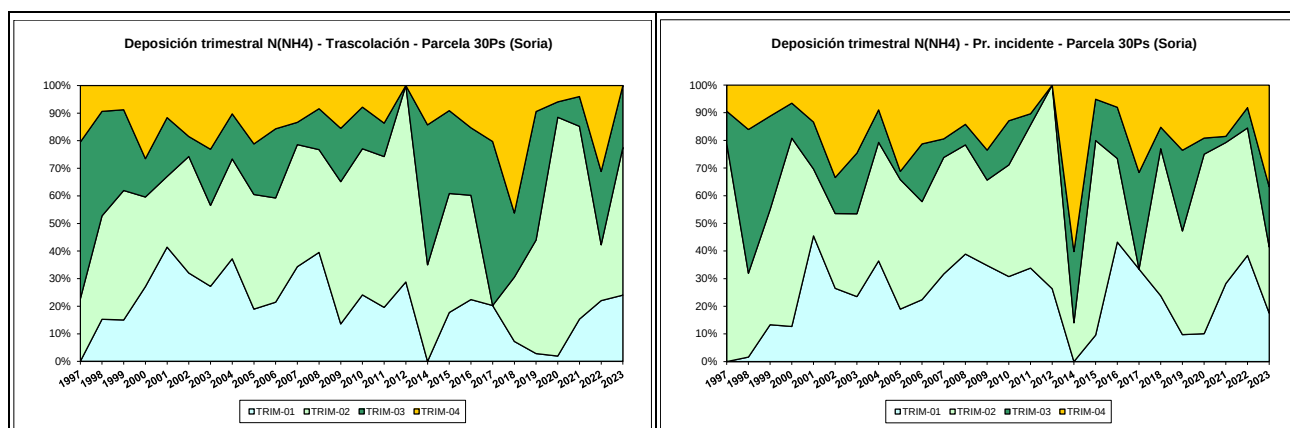
FIG 14: Variación temporal de deposición de amonio, diferencia TR-PI, porcentaje de deposición por trimestres
