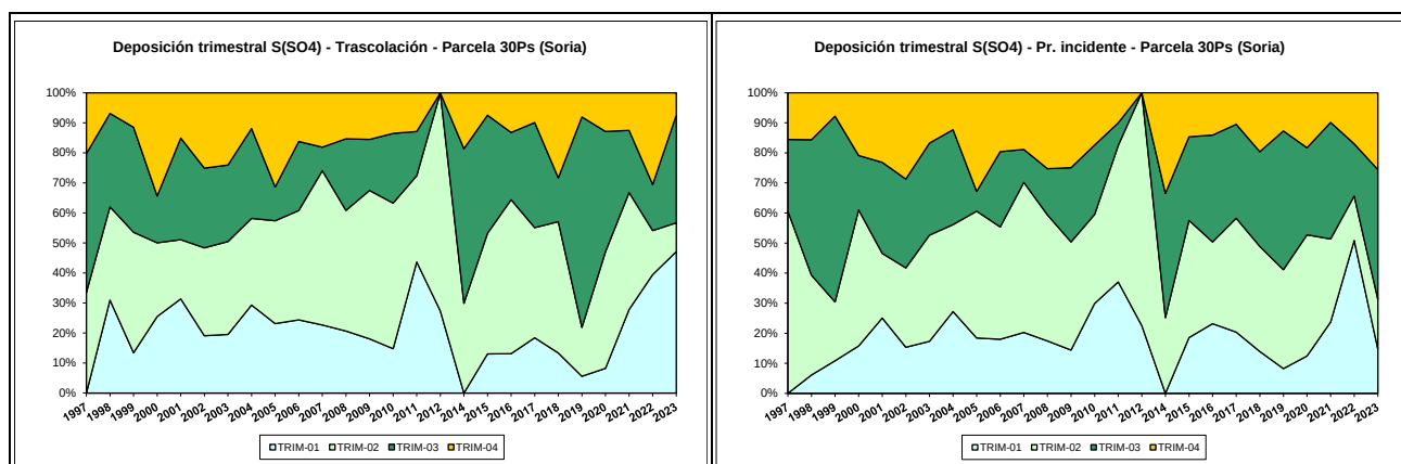
FIG 17: Variación temporal de deposición de sulfatos, diferencia TR-PI, porcentaje de deposición por trimestres
