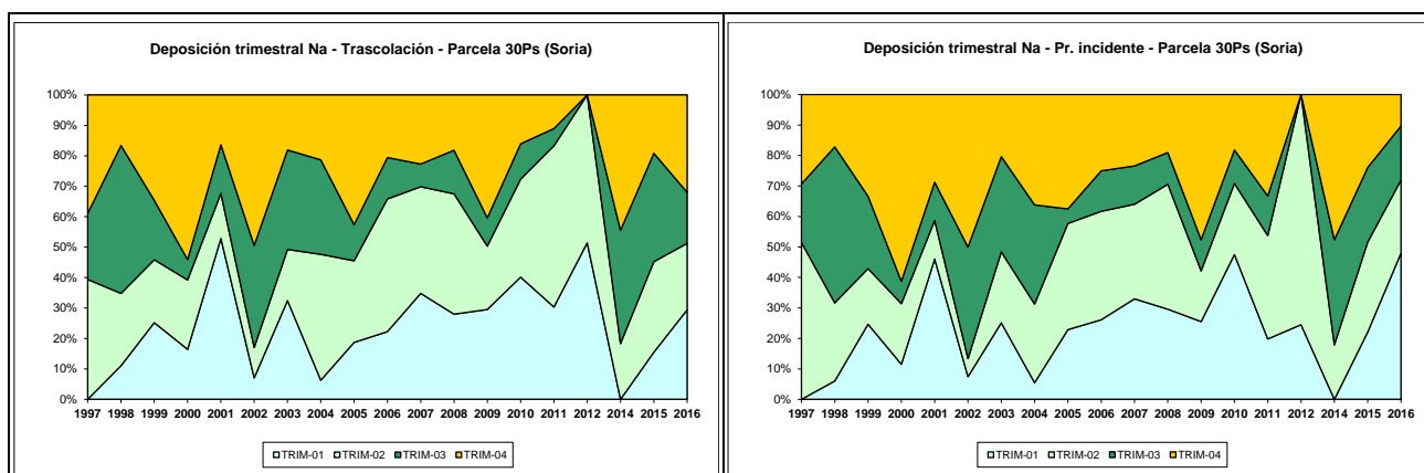
FIG 13: Variación temporal de deposición de Na, diferencia TR-PI, porcentaje de deposición por trimestres
