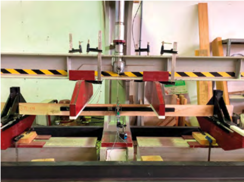
Foto. Fundación Cesefor. Ensayo a flexión de acuerdo con la norma UNE-EN 408
