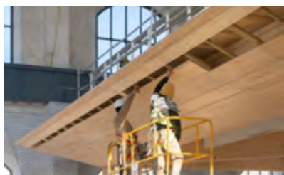
Foto. Rubén Pérez Bescós. Montaje de entablado de madera
