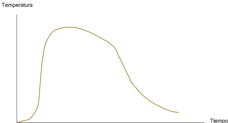
Figura 3. Curva tiempo-temperatura de un incendio real.
