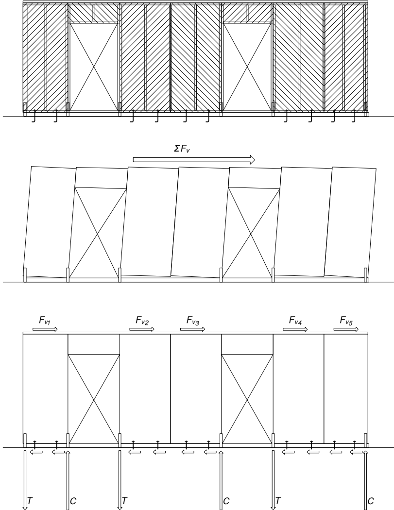
Figura 11. Muro compuesto de varios paneles.
