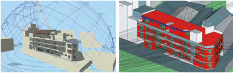
Simulación energética. Design Builder (izquierda) y DesignPH-PHPP (derecha). Foto: Daniel Pascual / sAtt Arquitectura Triple Balance.
