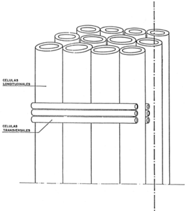
Figura 3. Esquema mecánico simplificado de la madera.
