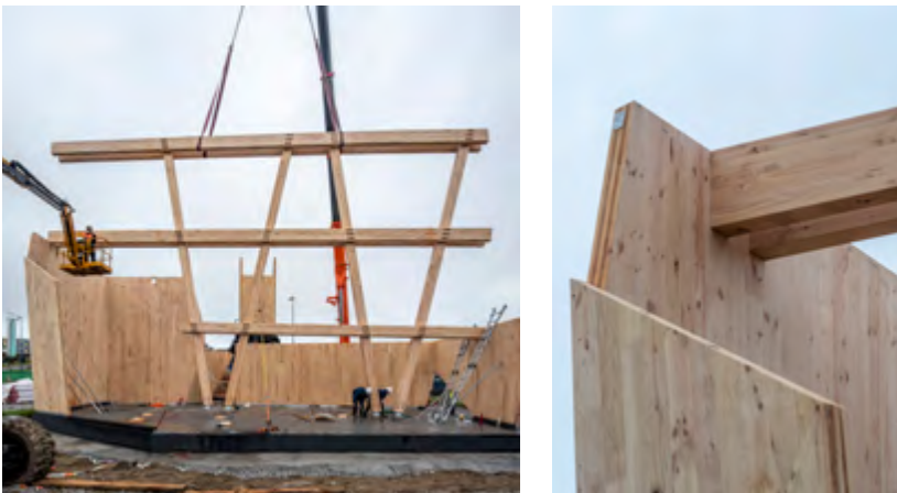
Figura 9: Colocación del pórtico mediante izado (izq.) y detalle de apoyo sobre el muro de fachada (dcha.). Fotografías: Héctor Santos-Díez.
