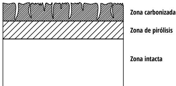
Figura 4. Cambios en la madera por la acción del fuego.
