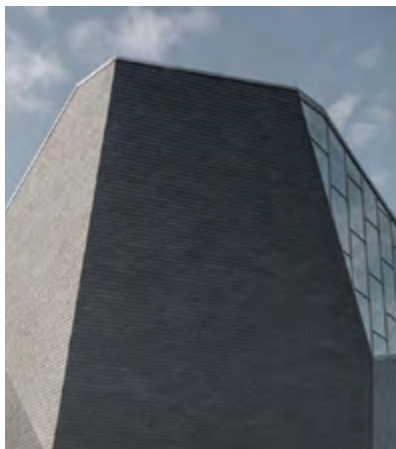
Figura 8: Fachada ventilada de pizarra. Detalle durante el montaje (izq.) y aspecto exterior del edificio una vez terminada su colocación (dcha.). Fotografías: Héctor Santos-Díez.
