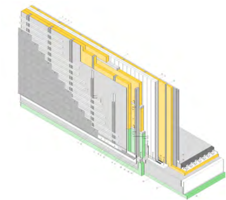
Figura 7: Solución constructiva de fachada.
