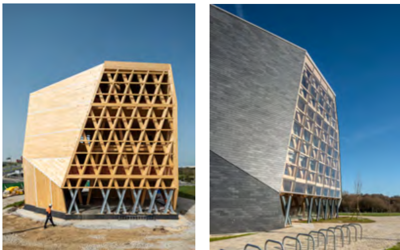
Figura 1: Edificio Impulso Verde. Vista exterior tras finalizar el montaje de la estructura (izq.) y tras la finalización de la urbanización (dcha.). Fotografías: Héctor Santos-Díez.
