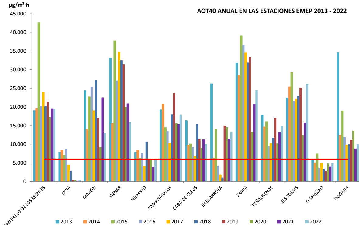
Figura 6. AOT40 anual en todas las estaciones de la red (2013 – 2022)
