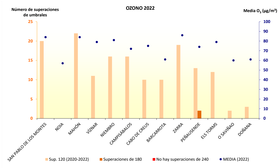
Figura 4. Media anual de O 3 en 2022, número de superaciones del máximo diario móvil octohorario (120 µg/m 3 ) en el periodo 2020-2022
