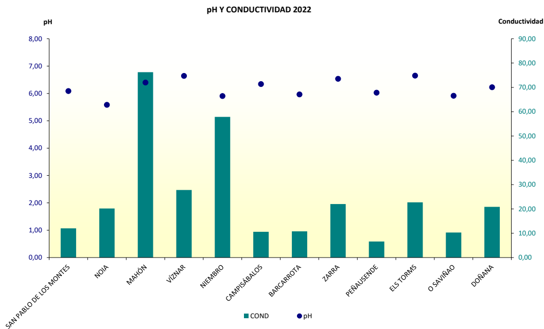
Figura 12. Media anual (ponderada con la precipitación) de pH y de conductividad en el año 2022
