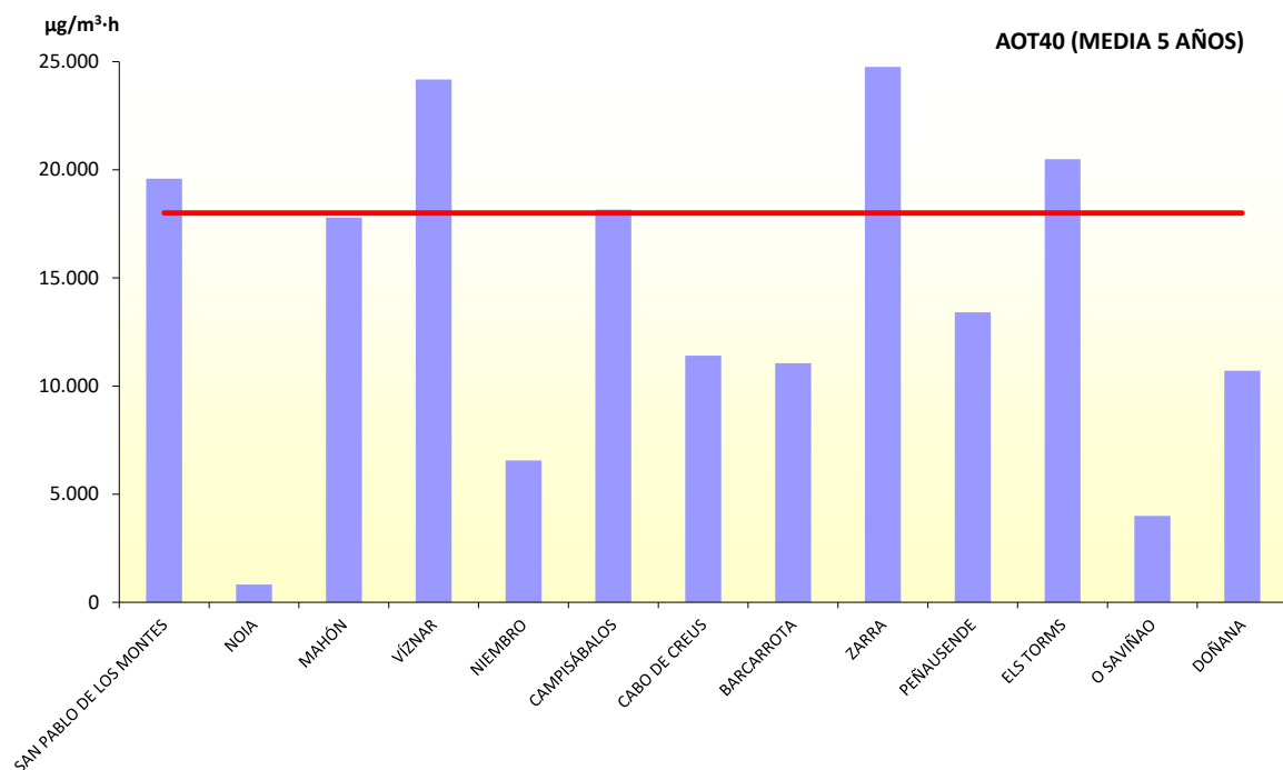
Figura 5. AOT40 (media de 5 años) en todas las estaciones de la red 2018-2022
