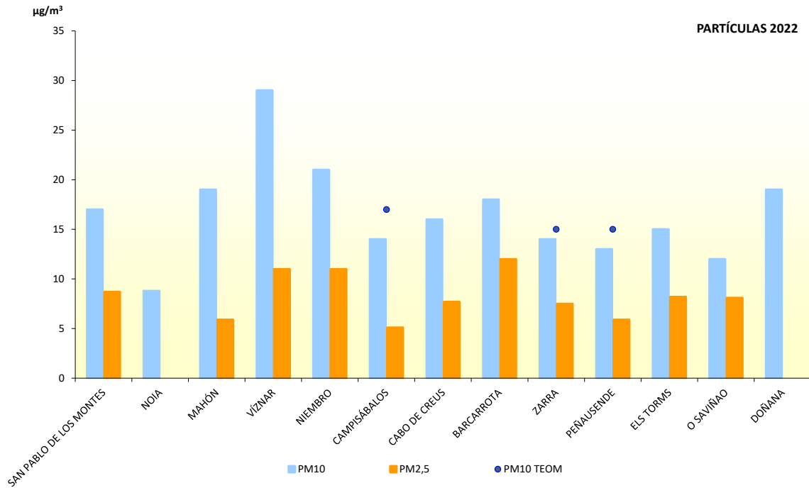
Figura 7. Datos medios anuales de partículas en 2022
