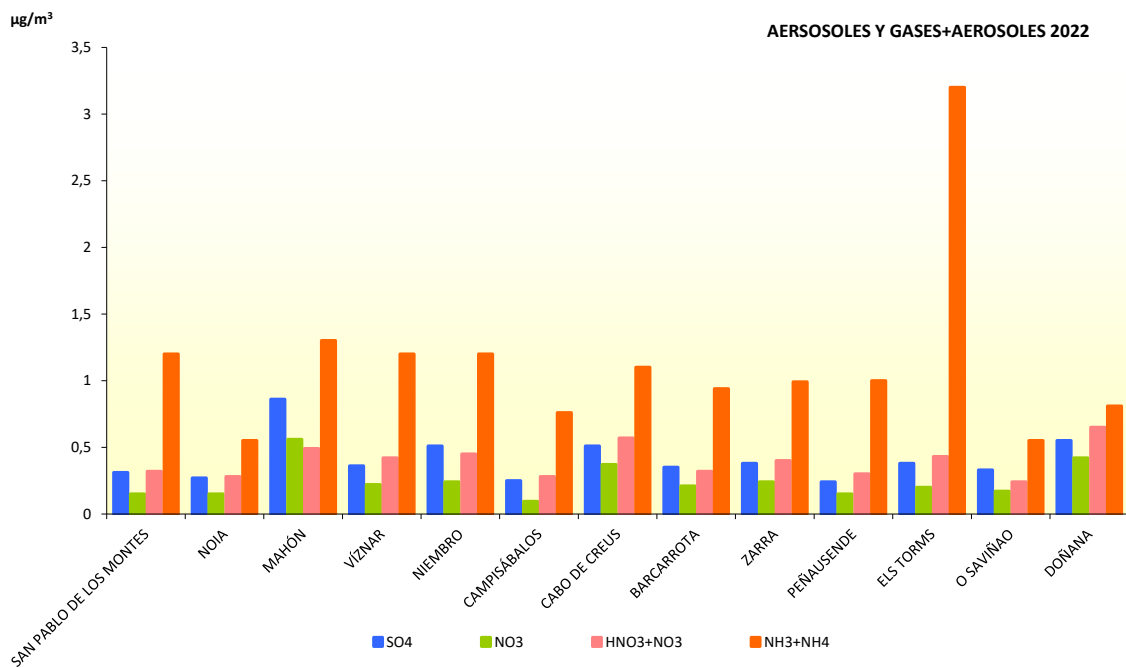
Figura 8. Datos medios anuales de aerosoles y gases + aerosoles en 2022
