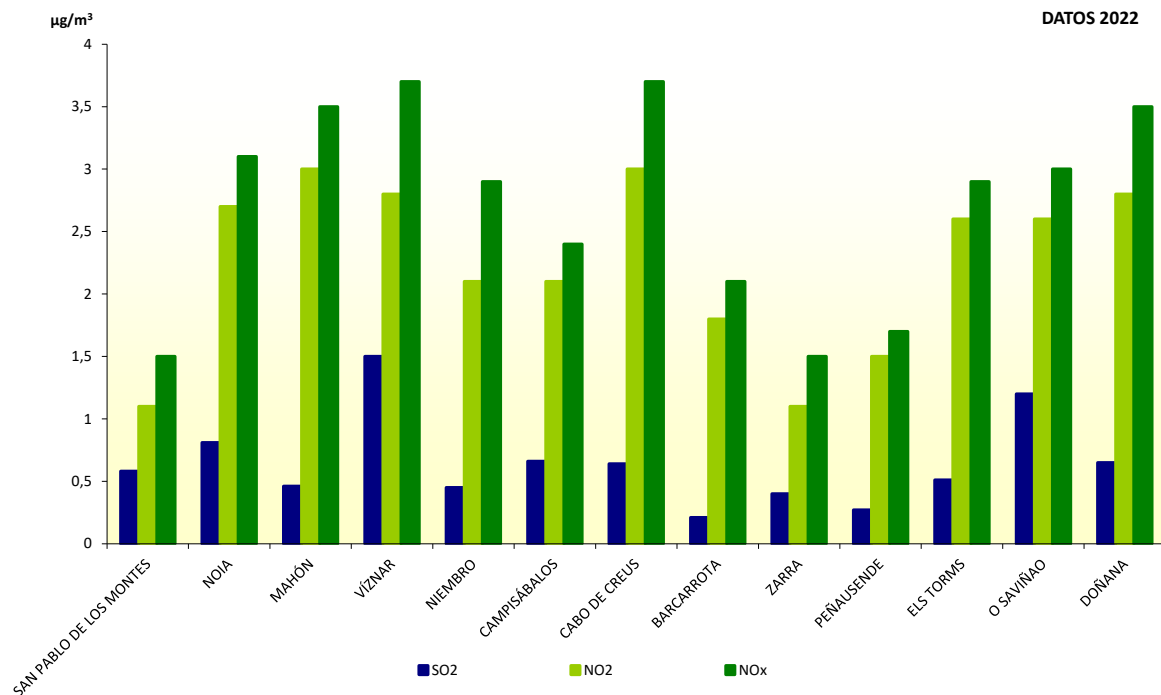
Figura 3. Datos de SO 2 , NO 2 y NO x en el año 2022
