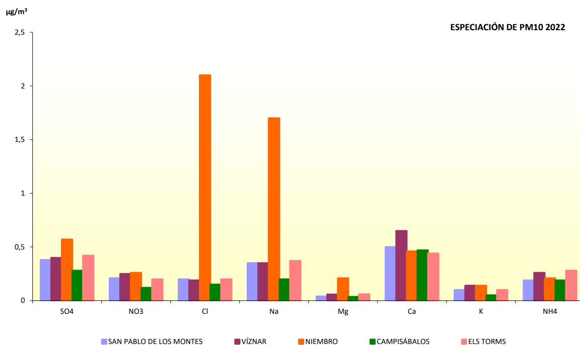
Figura 9. Datos medios anuales de especiación de PM10 en 2022
