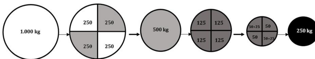
Figura 2. Esquema de la separación por cuarteos y obtención de la muestra.
