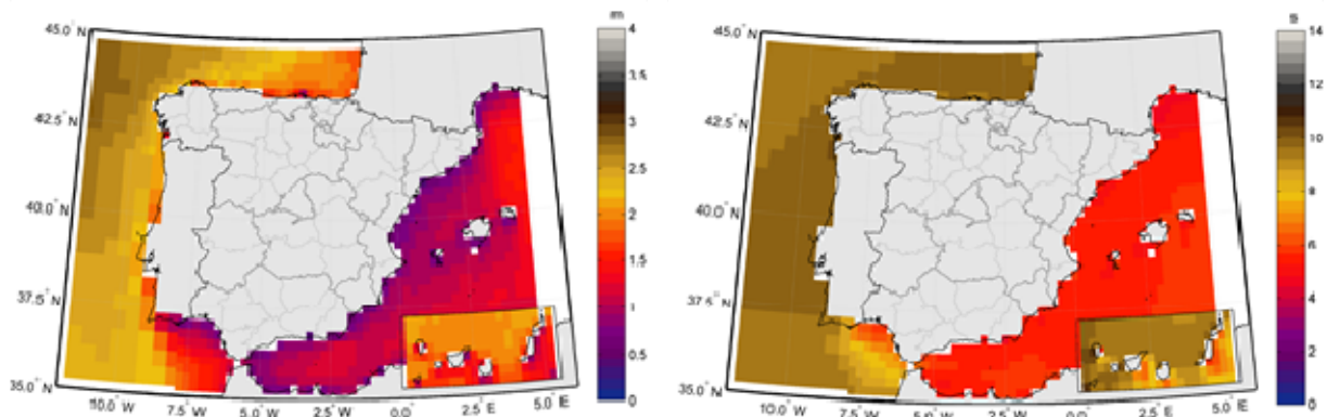
Figura 15. Altura de ola media anual en profundidades indefinidas en el entorno español (izquierda) y período de pico medio en profundidades indefinidas en el entorno español (derecha). Fuente: IHCantabria.
