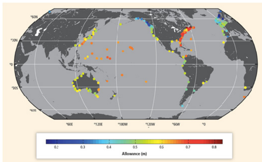
Figura 9. Incremento en la altura de las defensas de protección frente a inundación costera que sería necesario en el periodo 2081-2010 para preservar la misma frecuencia de excedencias experimentada en el periodo 1986-2005. El resultado se muestra para la localización de 182 mareógrafos y considerando las proyecciones regionales de aumento del mar relativo correspondientes al RCP4.5. (Fuente: Wong et al. 2013).
