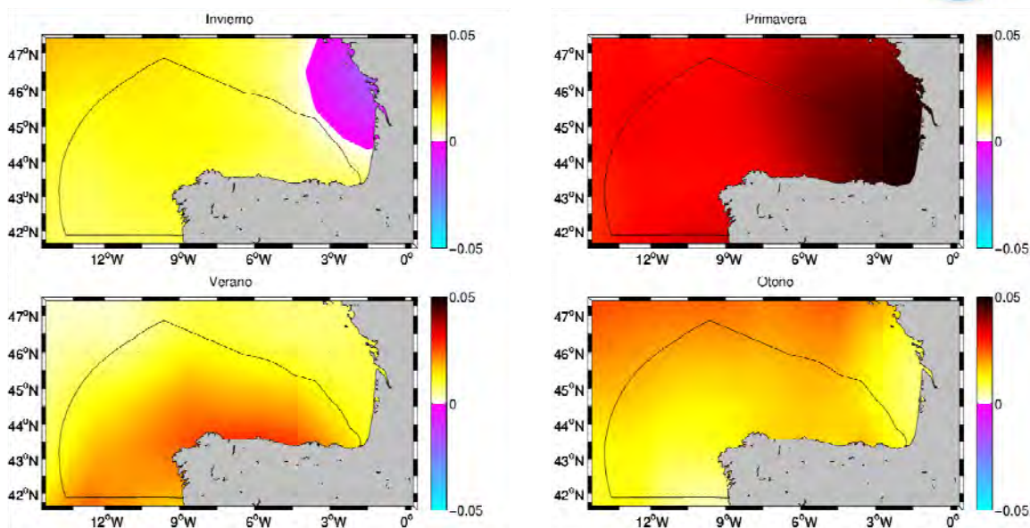
Figura 7.2. Tendencia de la SST por estaciones en la DM Noratlántica. El registro de reconstrucción SST de la NOAA (Reynolds et al. , 2002) que ofrece datos semanales en una malla de 1x1 desde principios de los 80.
