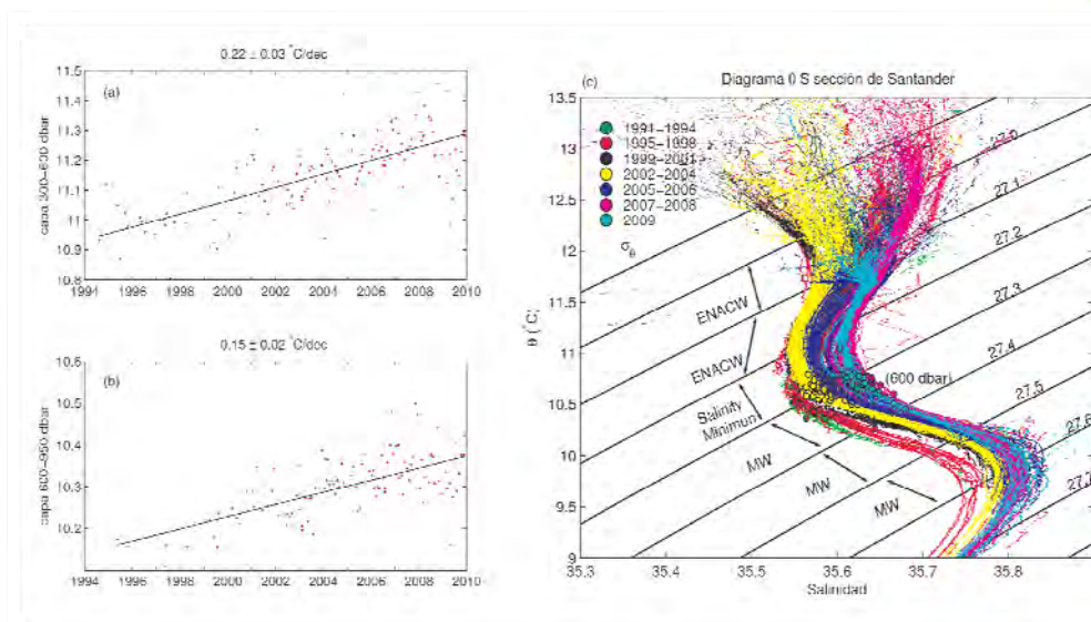
Figura 7.3. (a) Evolución de la temperatura en la estación 7 del Radial de Santander en las capas representativas de las aguas centrales (300–600 dbar) y (b) de la parte superior del agua mediterránea (600–950 dbar). (c) Evolución del diagrama \theta S distinguiendo diferentes periodos por medio de colores. Tomado de González-Pola et al. , 2012.
