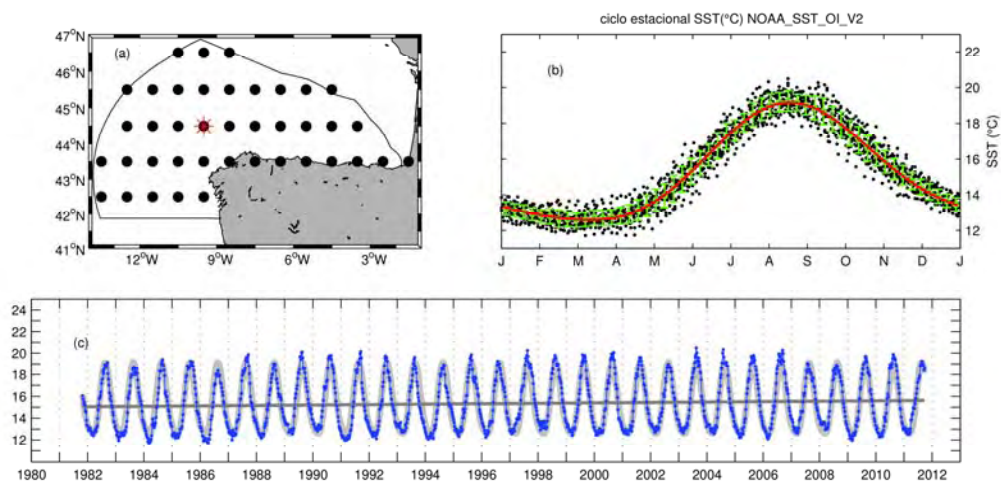
Figura 7.1. Ciclo estacional (b) y variabilidad interanual (c) de la SST en un punto representativo de la Demarcación Noratlántica (a). El registro reconstrucción SST de la NOAA (Reynolds et al. , 2002) que ofrece datos semanales en una malla de 1x1 desde principios de los 80.
