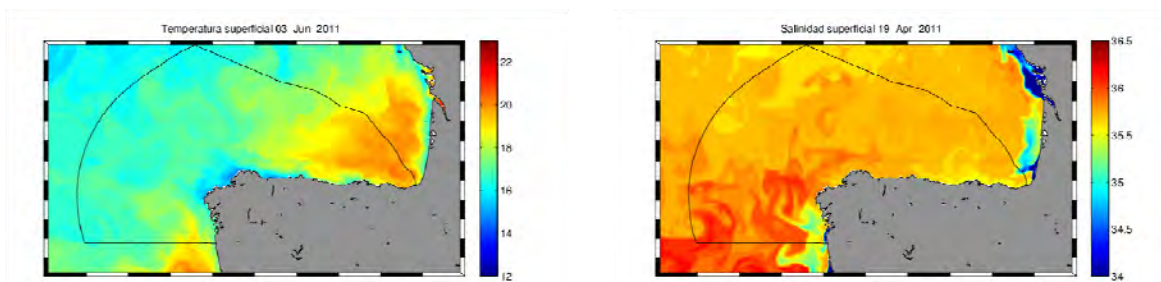
Figura 7.4. Salidas del sistema de predicción operacional MyOcean ( www.myocean.eu ) a) SST; b) SSS.
