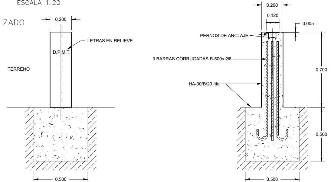
HITO DE HORMIGON TIPO II ESCALA 1:20
