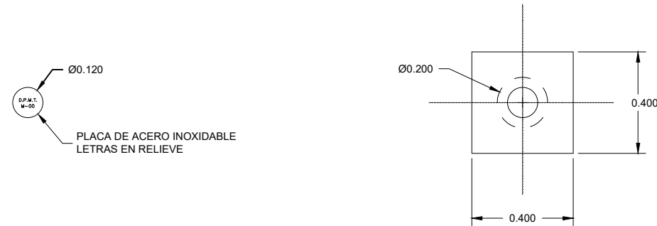
PLACA DE ACERO TIPO III ESCALA 1:10
