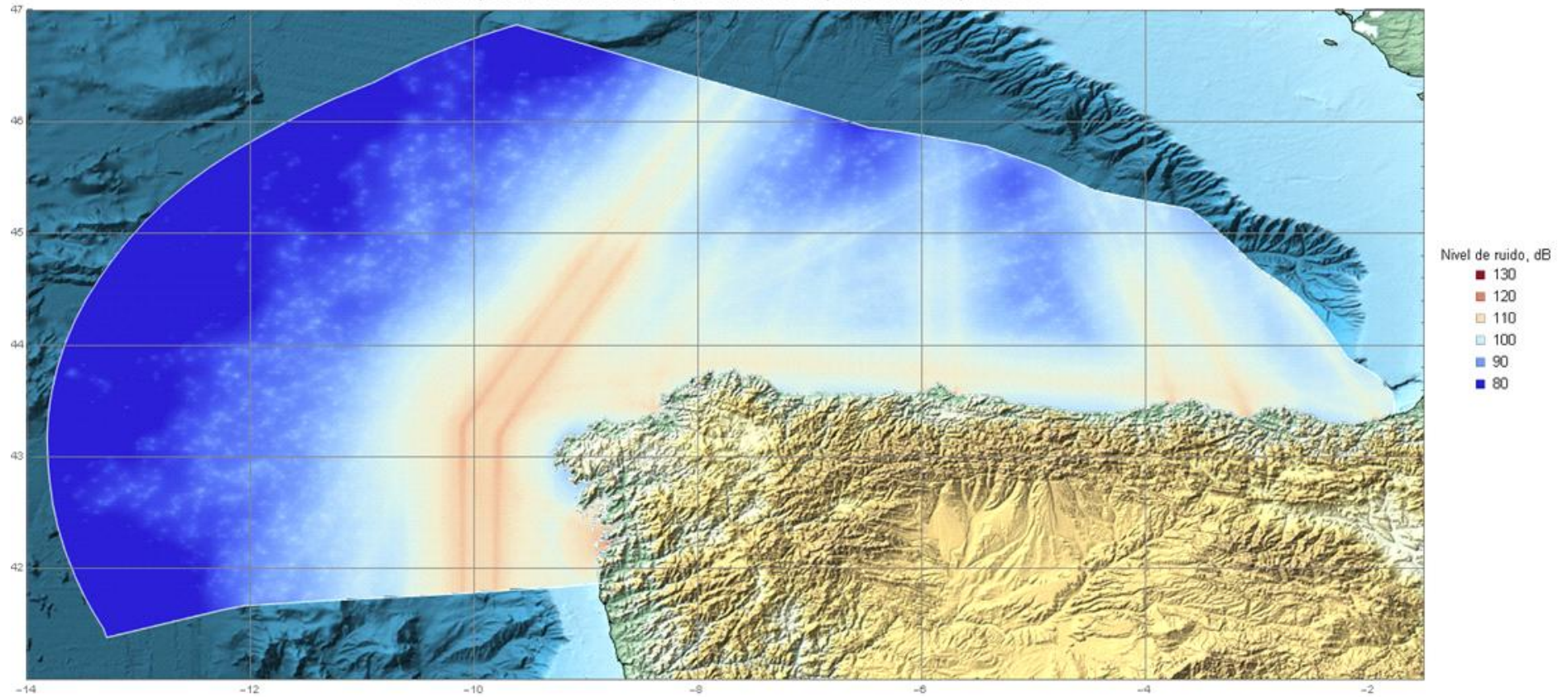
Figura 84. Niveles medio de ruido recibido dB re 1 \mu Pa en otoño de 2016, 63 Hz
