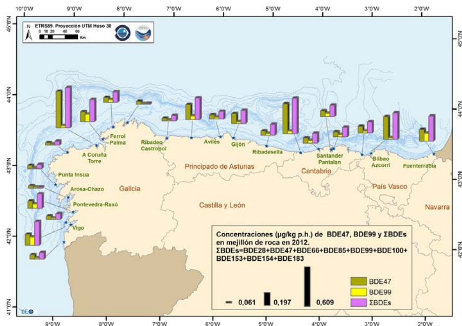
Figura 61. Distribución de la concentración de BDE47, BDE99 y \Sigma\text{BDEs} ( \mu\text{g}/\text{kg p.h.} ) en mejillón de roca a lo largo de la costa de la DM noratlántica (2012).
