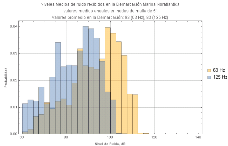
Figura 89. Porcentaje de niveles medio de ruido recibido dB re 1 \mu Pa anuales a 63 y 125 Hz en la DM noratlántica
