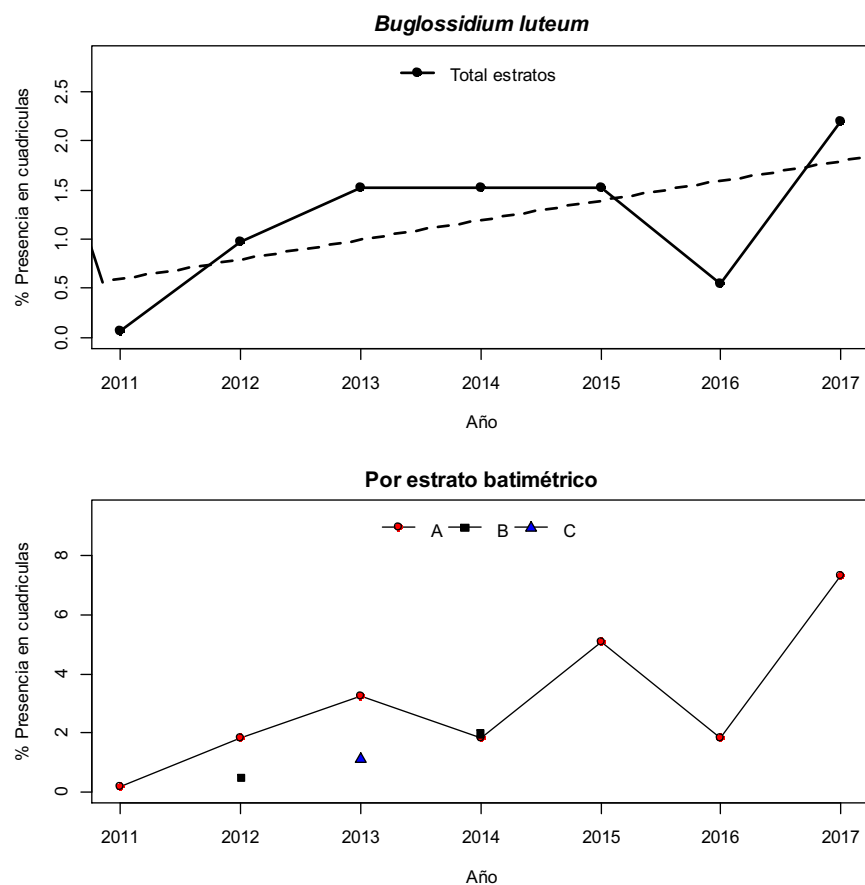
Figura 21. En la parte superior: patrón de distribución espacial de Buglossidium luteum desde 2011 a 2017, los puntos indican el porcentaje de cuadrículas con presencia. La línea discontinua indica la tendencia temporal del porcentaje del número de cuadrículas con presencia obtenida con un modelo lineal. En la parte inferior: patrón de distribución espacial de la especie en función de los distintos estratos batimétricos estudiados (A =70-120 m, B = 121-200 m, C = 201-500 m).
