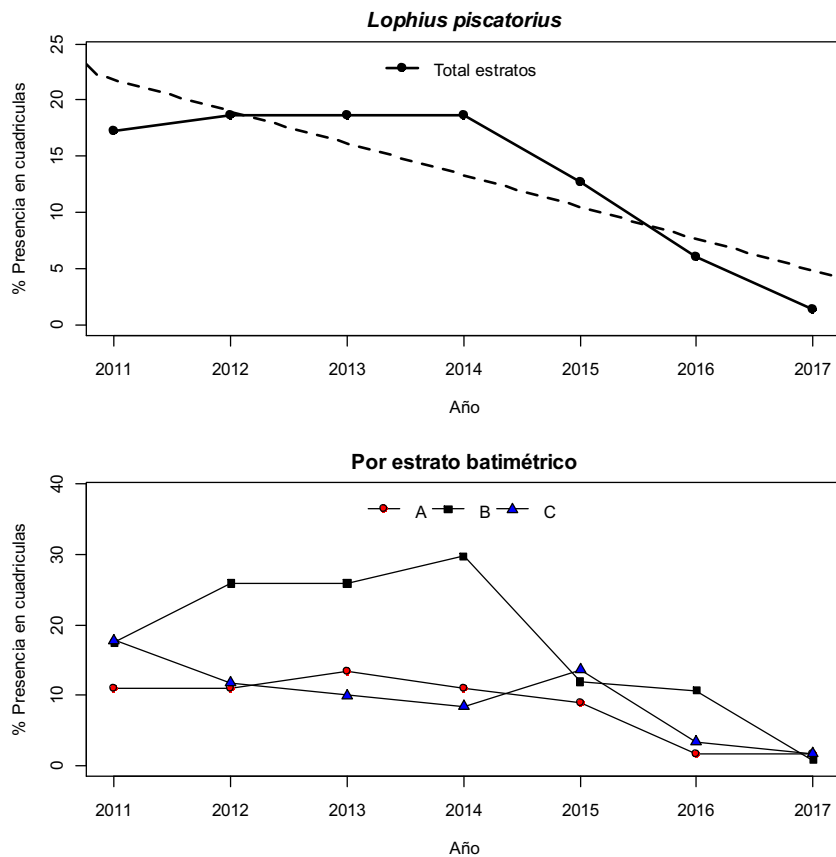
Figura 24. En la parte superior: patrón de distribución espacial de Lophius piscatorius desde 2011 a 2017, los puntos indican el porcentaje de cuadrículas con presencia. La línea discontinua indica la tendencia temporal del porcentaje del número de cuadrículas con presencia obtenida con un modelo lineal. En la parte inferior: patrón de distribución espacial de la especie en función de los distintos estratos batimétricos estudiados (A = 70-120 m, B = 121-200 m, C = 201-500 m).
