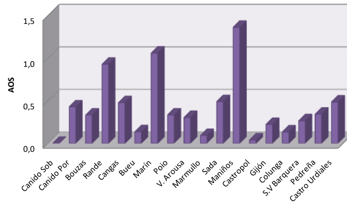
Figura 66. Índice del estado del oviducto (AOS) en poblaciones de Nassarius reticulatus de la DM noratlántica en 2014-2015.
