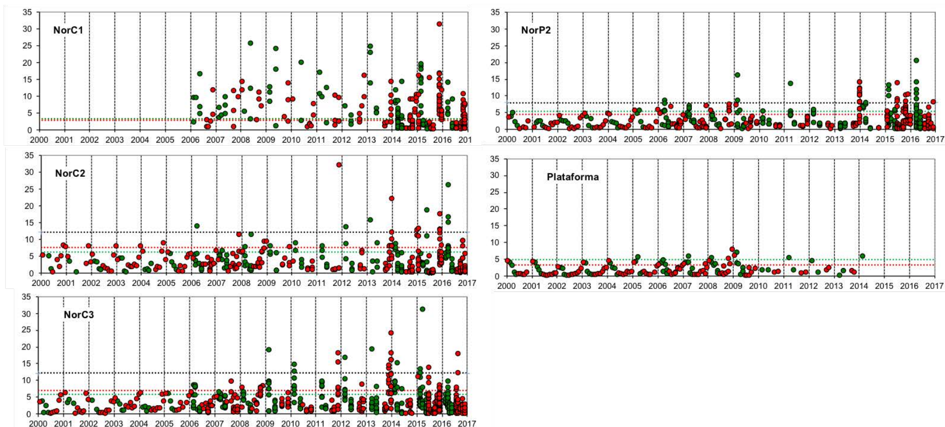
Figura 37. Concentración de nitrato obtenida en las áreas de productividad de la DM noratlántica. En verde se indican los valores obtenidos durante el periodo considerado más productivo del año (febrero, marzo, abril y mayo) y en rojo los obtenidos durante el resto del ciclo anual. Los datos correspondientes al período 2011-2016 son los proporcionados por las comunidades autónomas, generados desde los programas de seguimiento de la DMA. Las líneas horizontales indican los valores límite del BEA para la condición Bueno/Moderado establecidos para la DMA (línea negra) y los valores de base de las Estrategias Marinas determinados en la evaluación inicial (periodo productivo en verde y resto del año en rojo). Nota: los valores bases para el área NorC1 corresponden al Percentil 90 (P90) calculado para el periodo del que se disponen datos (2006-2016).
