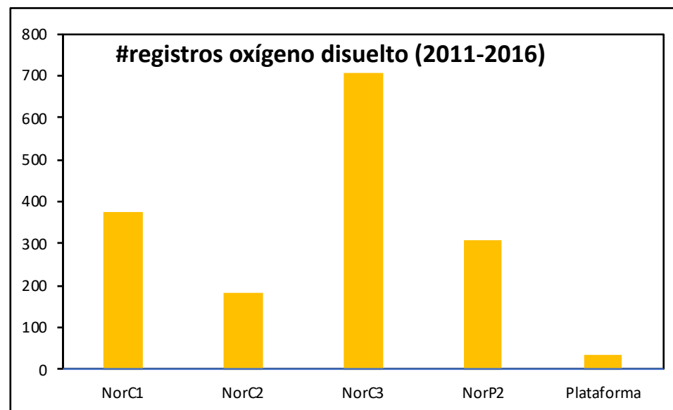
Figura 42. Registros de concentración de oxígeno en 2011-2016, recopilados para la presente evaluación inicial
