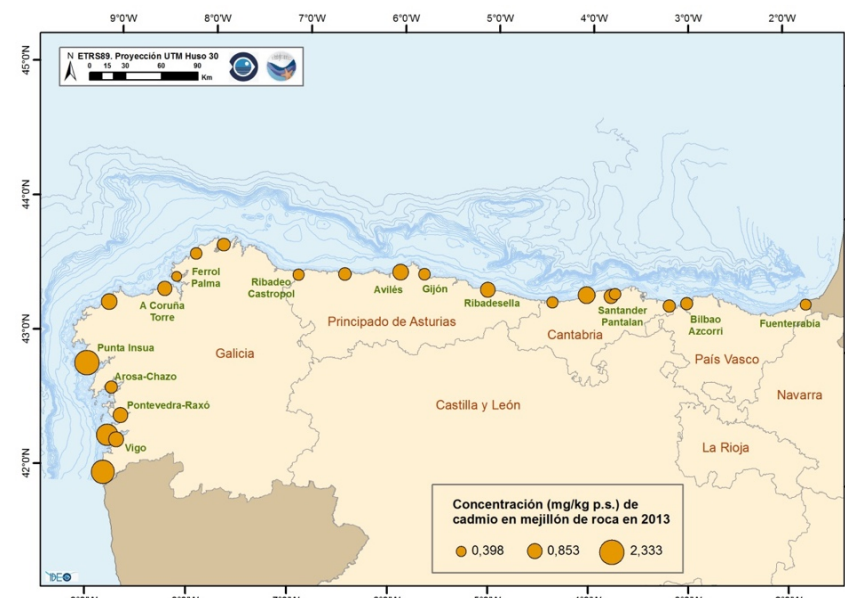
Figura 50. Distribución de la concentración de cadmio (mg/kg p.s.) en mejillón de roca a lo largo de la costa de la DM noratlántica (2013).
