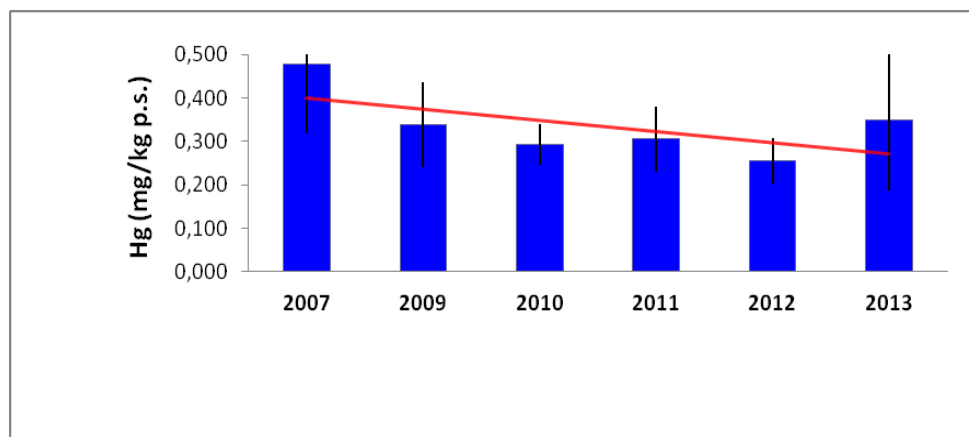
Figura 54. Concentraciones de mercurio en músculo de merluza ( Merluccius merluccius ) del Cantábrico. 2007-2013 Los niveles de Hg son superiores en las muestras de merluza procedentes del Cantábrico que en las de Galicia.
