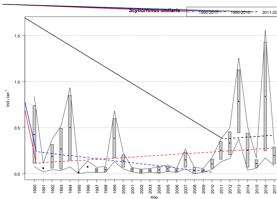
Figura 16. Evolución de los rendimientos de Scyliorhinus stellaris entre los años 1990 y 2017. Las líneas indican la tendencia calculada usando un modelo lineal. Roja: 1990-2017, Azul: 1990-2010, Negra: 2011-2017.
