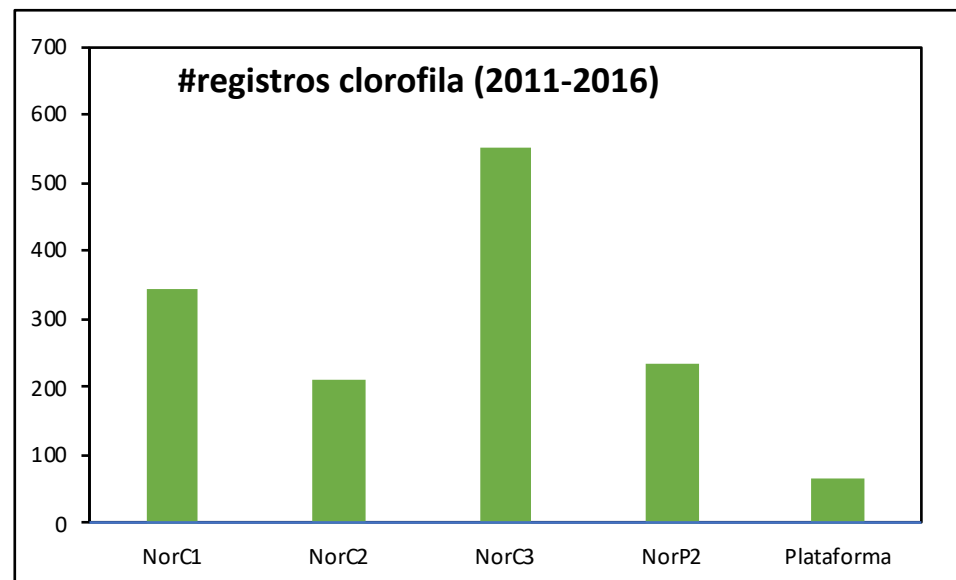
Figura 40.Registros de clorofila recopilados para la evaluación del criterio D5C2.
