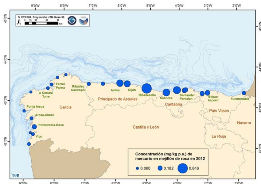
Figura 47. Distribución de la concentración de mercurio (mg/kg p.s.) en mejillón de roca a lo largo de la costa de la DM noratlántica (2012).
