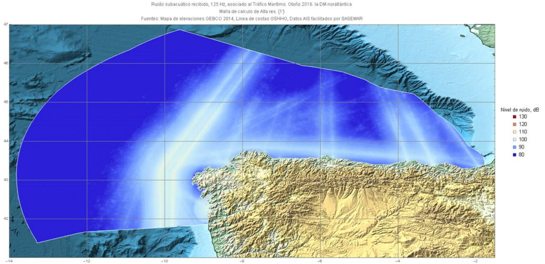
Figura 88. Niveles medio de ruido recibido dB re 1 \mu Pa en otoño de 2016, 125 Hz
