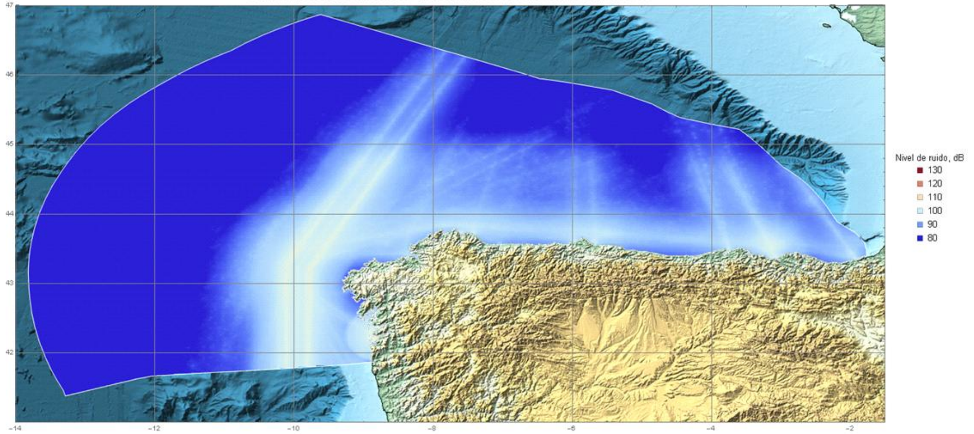
Figura 85. Niveles medio de ruido recibido dB re 1 \mu Pa en invierno de 2016, 125 Hz
