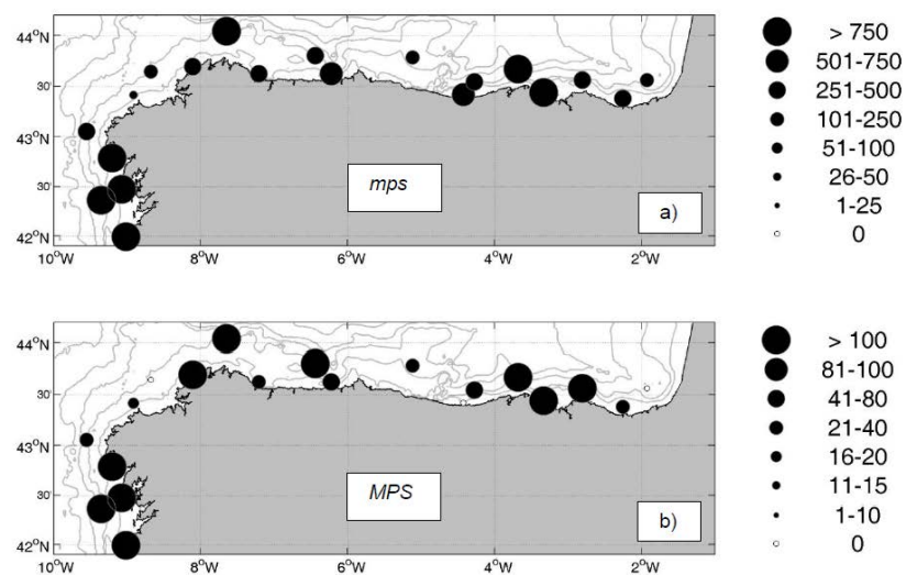
Figura 76. Microplásticos y macroplásticos en aguas superficiales durante la primavera de 2014.
