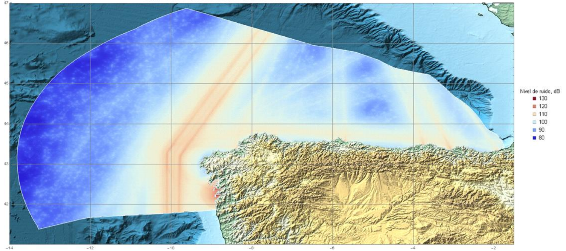
Figura 83. Niveles medio de ruido recibido dB re 1 \mu Pa en verano de 2016, 63 Hz
