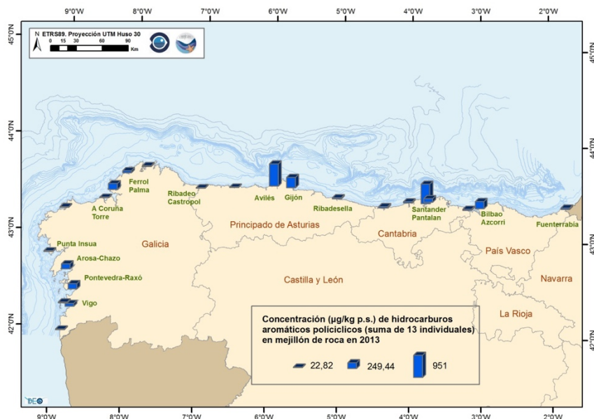
Figura 55. Distribución de la concentración total (suma de 13 PAHs individuales) de hidrocarburos aromáticos policíclicos ( \mu\text{g}/\text{kg p.s.} ) en mejillón de roca a lo largo de la costa de la DM noratlántica (2012).
