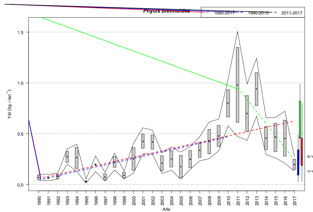
Figura 15. Evolución de los rendimientos de Phycis blennoides entre los años 1990 y 2017. Las líneas indican la tendencia calculada usando un modelo lineal. Roja: 1990-2017, Azul: 1990-2010, Verde: 2011-2017.
