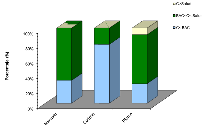
Figura 44. Distribución de concentración (C) de Hg, Cd y Pb en mejillón (expresada en porcentaje respecto al total de muestras de la distribución espacial 2013) según los criterios de evaluación propuestos.
