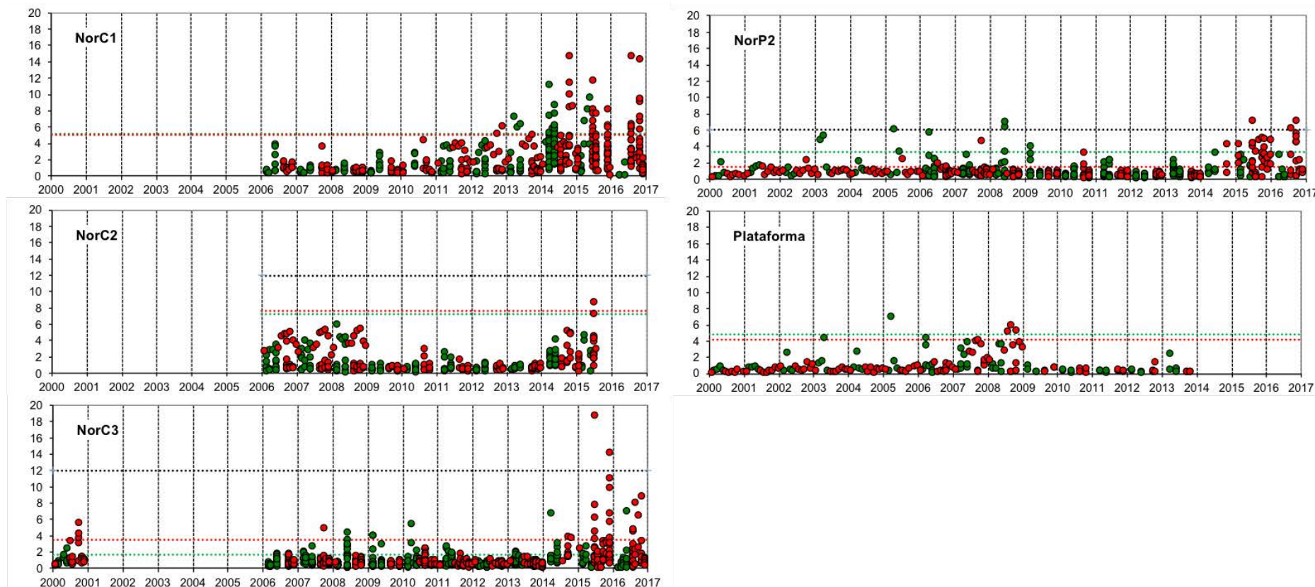
Figura 41. Concentración de clorofila a obtenida en las áreas de productividad de la DM noratlántica. En verde se indican los valores obtenidos durante el periodo considerado más productivo del año (febrero, marzo, abril y mayo) y en rojo los obtenidos durante el resto del ciclo anual. Los datos correspondientes al periodo 2011-2016 son los proporcionados por las comunidades autónomas, generados desde los programas de seguimiento de la DMA. Las líneas horizontales indican los valores de referencia de la DMA (línea negra) y los valores de base de las Estrategias Marinas (periodo productivo en verde y resto del año en rojo). Nota: los valores bases para el área NorC1 corresponden al Percentil 90 (P90) calculado para el periodo del que se disponen datos (2006-2016).
