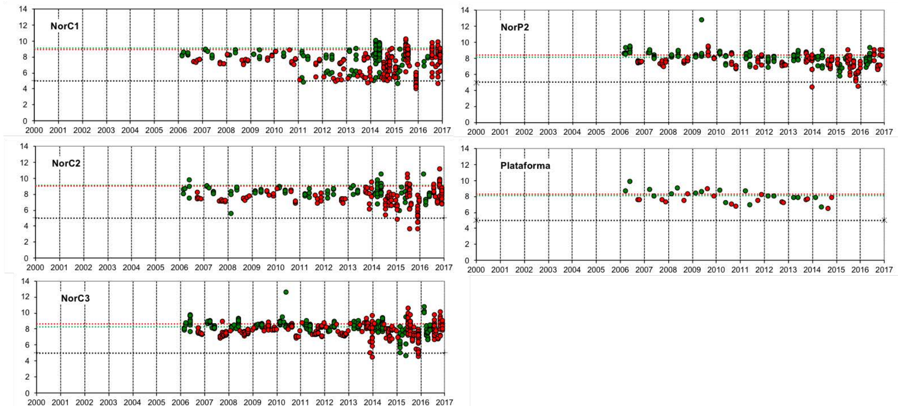
Figura 43. Concentración de oxígeno obtenida en las áreas de productividad de la Demarcación Noratlántica. En verde se indican los valores obtenidos durante el periodo considerado más productivo del año (febrero, marzo, abril y mayo) y en rojo los obtenidos durante el resto del ciclo anual. Los datos correspondientes al periodo 2011-2016 son los proporcionados por las comunidades autónomas, generados desde los programas de seguimiento de la DMA. Las líneas horizontales indican la línea horizontal indica el valor umbral (5 \text{mg/l} ) (línea negra) y los valores de base de las Estrategias Marinas (periodo productivo en verde y resto del año en rojo).
