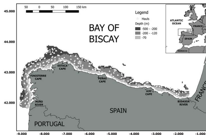
Figura 26.- Mapa de área de estudio que muestra la posición de los lances (triángulos blancos) durante las campañas Demersales (2007-2010) en los tres estratos de profundidad: 70-120, 121-200, 201-500m.
