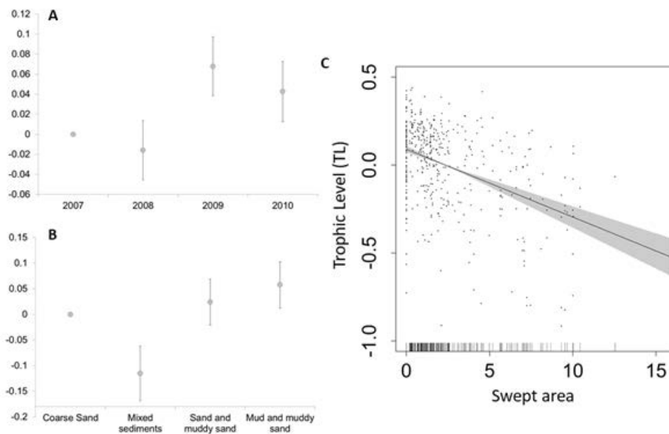
Figura 31. Resultados del Modelo Aditivo Generalizado (GAM) usando VMS, Profundidad y Tipo de sedimento como variables explicativas de los cambios observados en el indicador MTL2. Solo se muestran las variables que resultaron significativas.
