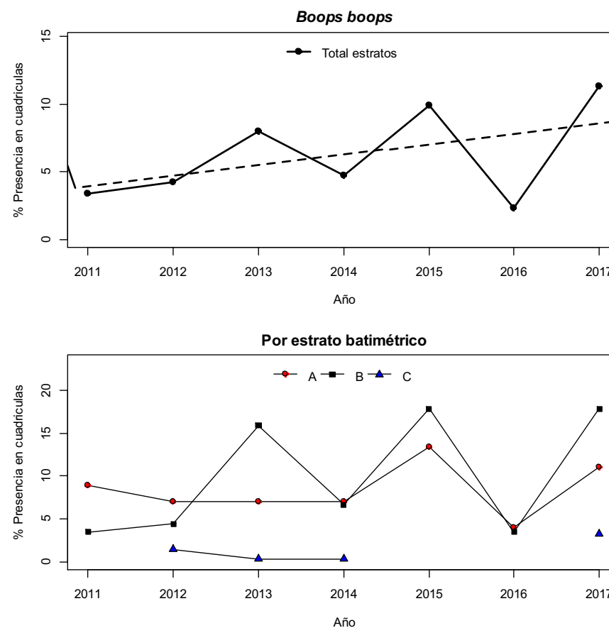
Figura 22. En la parte superior: patrón de distribución espacial de Boops boops desde 2011 a 2017, los puntos indican el porcentaje de cuadrículas con presencia. La línea discontinua indica la tendencia temporal del porcentaje del número de cuadrículas con presencia obtenida con un modelo lineal. En la parte inferior: patrón de distribución espacial de la especie en función de los distintos estratos batimétricos estudiados (A =70-120 m, B = 121-200 m, C = 201-500 m).
