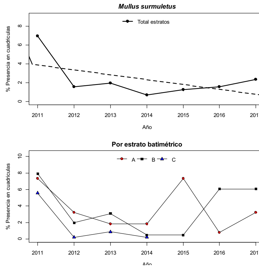
Figura 23. En la parte superior: patrón de distribución espacial de Mullus surmuletus desde 2011 a 2017, los puntos indican el porcentaje de cuadrículas con presencia. La línea discontinua indica la tendencia temporal del porcentaje del número de cuadrículas con presencia obtenida con un modelo lineal. En la parte inferior: patrón de distribución espacial de la especie en función de los distintos estratos batimétricos estudiados (A = 70-120 m, B = 121-200 m, C = 201-500 m).
