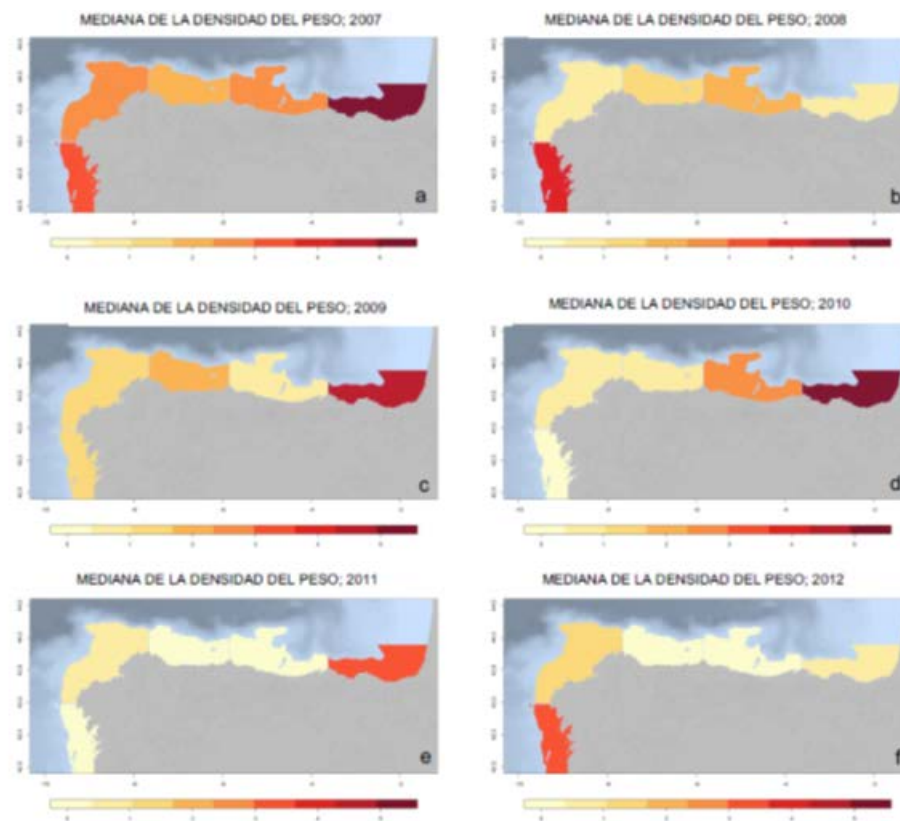
Figura 70. Mapas de variabilidad de la mediana ( \text{Kg}/\text{Km}^2 ) de la basura marina total por áreas y por años. Siendo a-2007; b-2008; c-2009 ; d-2010; e-2011 y f-2012
