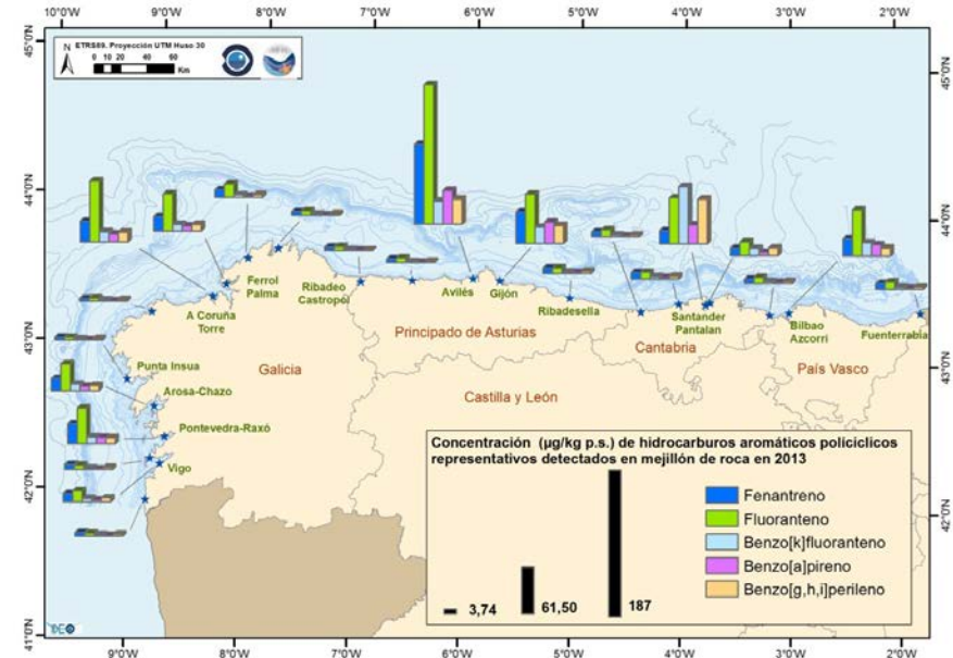
Figura 58. Distribución de la concentración de fenantreno, fluoranteno, benzo(k)fluoranteno, benzo(a)pireno y benzo(g,h,i)perileno ( \mu\text{g}/\text{kg p.s.} ) en mejillón de roca a lo largo de la costa de la DM noratlántica (2013).
