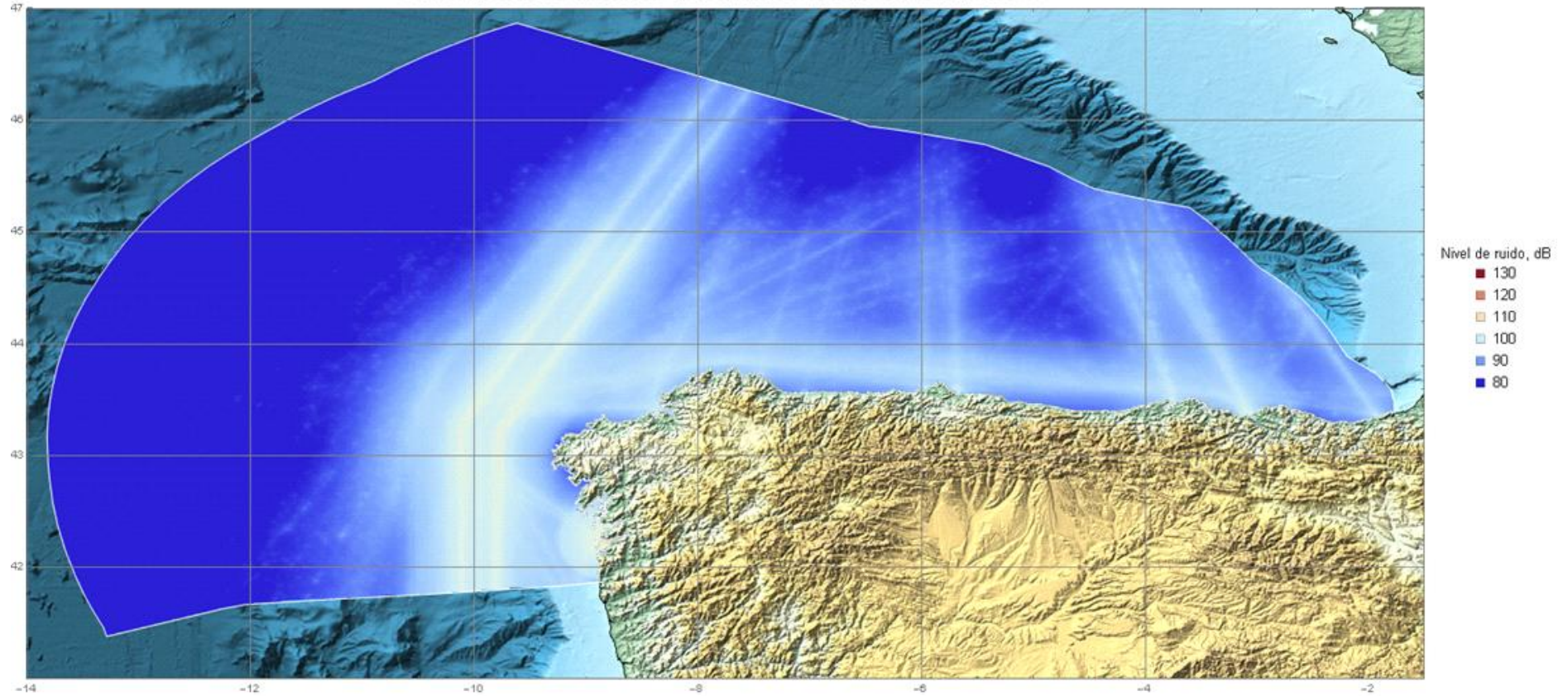
Figura 86. Niveles medio de ruido recibido dB re 1 \mu Pa en primavera de 2016, 125 Hz
