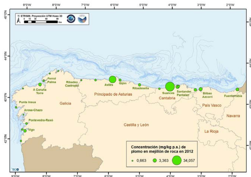
Figura 51. Distribución de la concentración de plomo (mg/kg p.s.) en mejillón de roca a lo largo de la costa de la DM noratlántica (2012).
