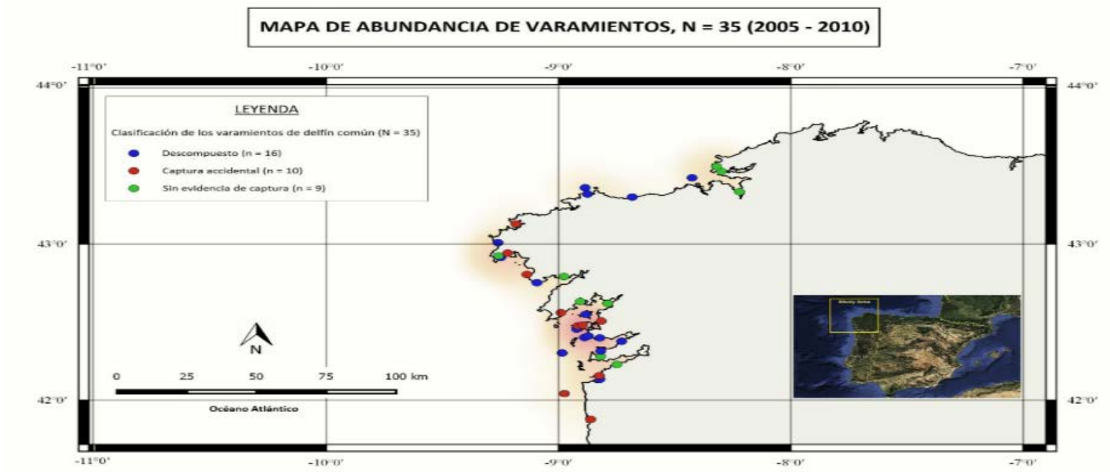
Figura 78. Mapa de abundancia de los varamientos de los 35 delfines comunes en la costa de Galicia (no de España) entre los años 2005 y 2010. Los puntos muestran la localización exacta de la costa gallega donde se encontraron los cuerpos de los individuos, en color rojo (●) los cadáveres que mostraban signos de captura accidental o enmalle, y en color verde (●) los cadáveres que no mostraban signos de captura o enmalle con las artes de pesca
