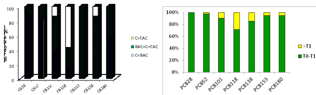
Figura 46. Distribución de concentración (C) de CB28, CB52, CB101, CB118, CB153, CB138 y CB180 (expresada en porcentaje respecto al total de muestras de la distribución espacial 2013) según los criterios de evaluación propuestos en a) mejillón (drch) y b) en merluza (izq)
