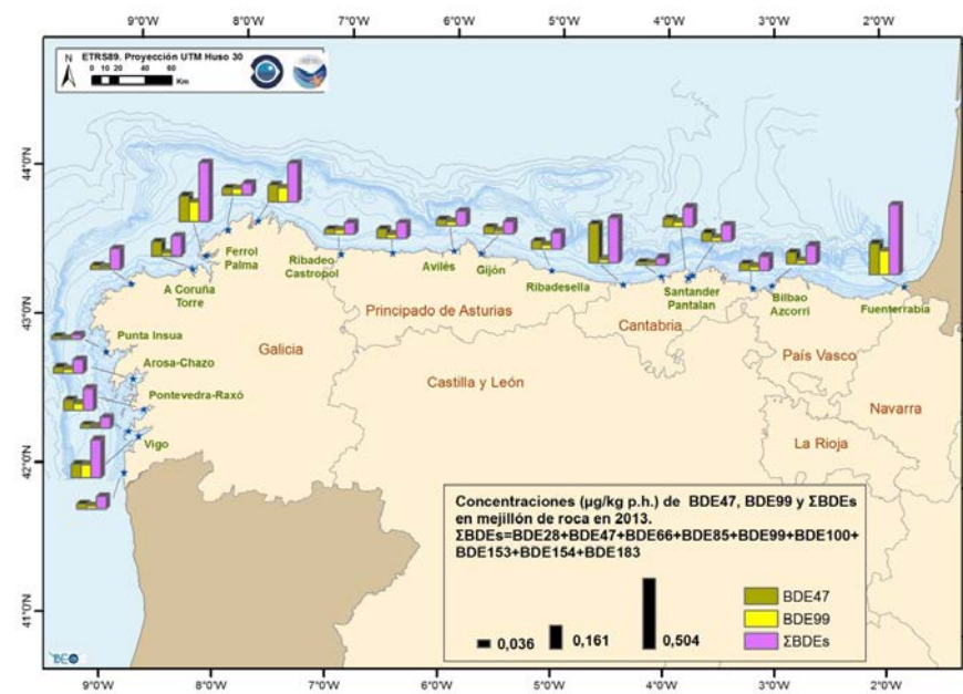
Figura 62. Distribución de la concentración de BDE47, BDE99 y \Sigma\text{BDEs} ( \mu\text{g}/\text{kg p.h.} ) en mejillón de roca a lo largo de la costa de la DM noratlántica (2013).
