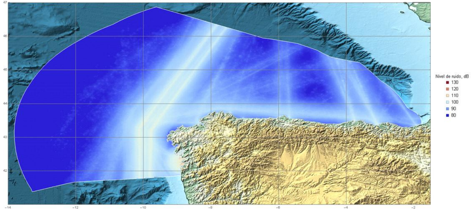
Figura 87. Niveles medio de ruido recibido dB re 1 \mu Pa en verano de 2016, 125 Hz
