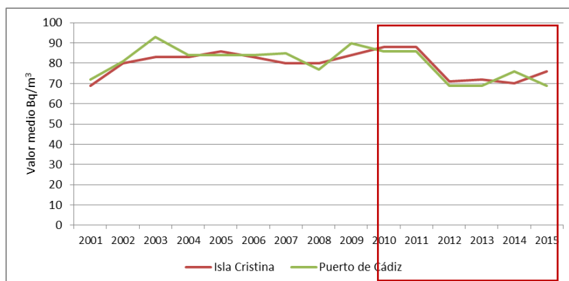
Figura 68. Concentración del índice de actividad alfa total ( Bq/m^3 ) en las estaciones de la demarcación
