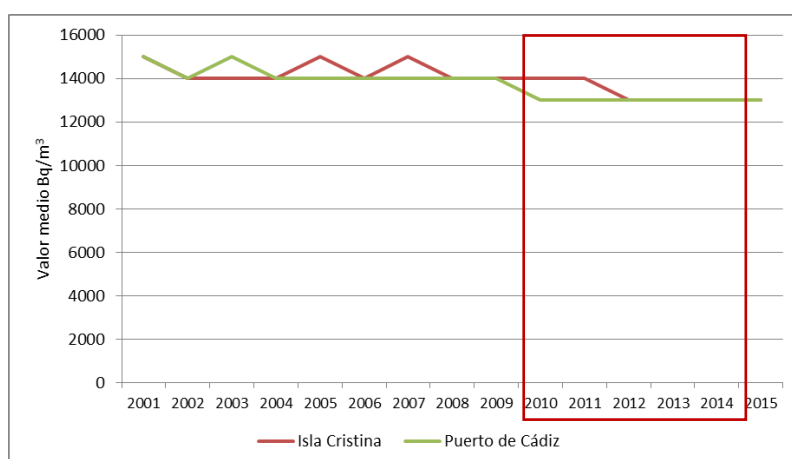
Figura 69. Concentración del índice de actividad beta total ( Bq/m^3 ) en las estaciones de la demarcación
