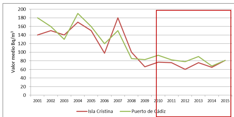
Figura 70. Concentración de actividad de tritio ( Bq/m^3 ) en las estaciones de la demarcación
