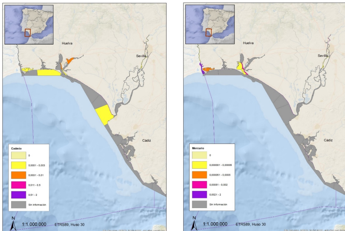
Figura 45. Aportes directos de cadmio (t/año, izquierda) y mercurio (t/año, derecha) por masa de agua costera o de transición
