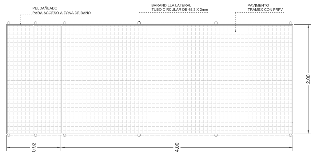
PLANTA e 1/40
